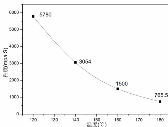
图1、热熔胶5160粘度随温度变化曲线
